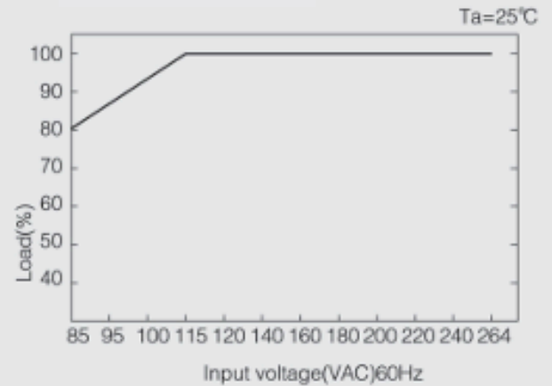
ıktı Gcnn Dşmesi VS Giriş Voltajı
