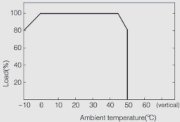
Derating Eđrisi
